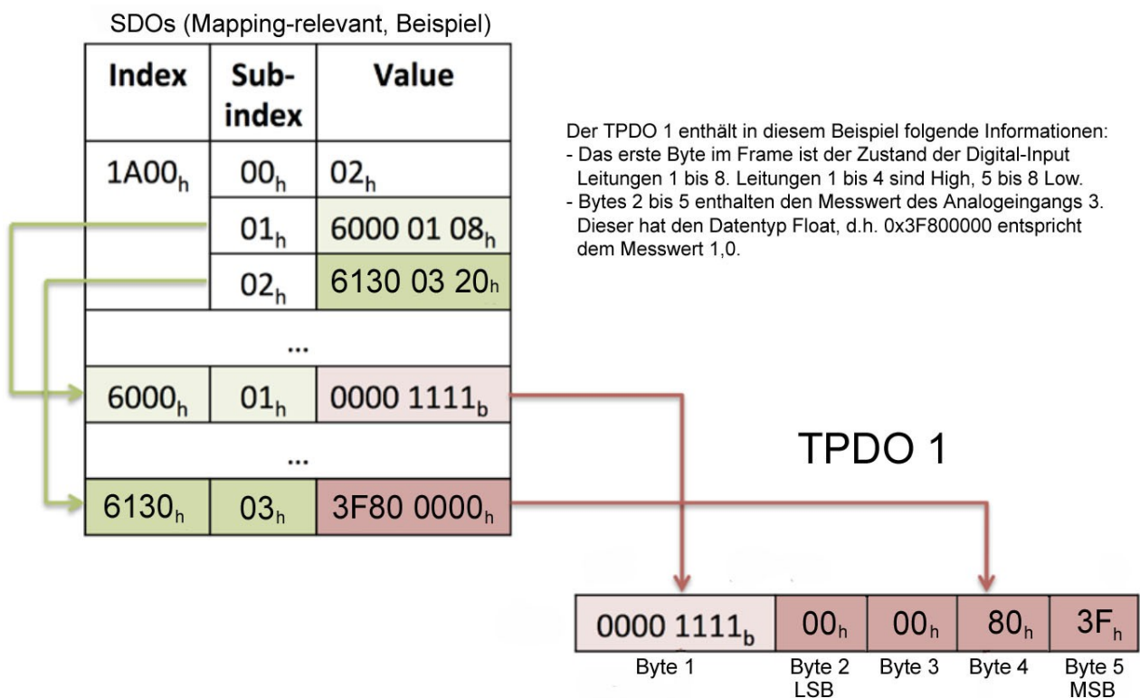
Abbildung 1: Beispiel für Mapping des TxPDO 1
